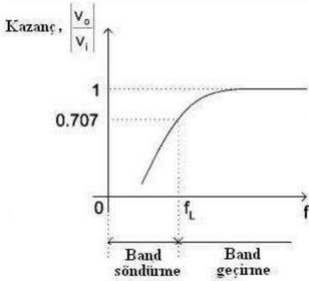
Şekil 1: Yüksek geçiren filtrenin kazanç/frekans grafiği
