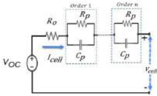
Şekil 3: n farklı RC Eşdeğer Devre Modeli
