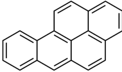
Şekil 2. Benzo(a)piren molekülü
