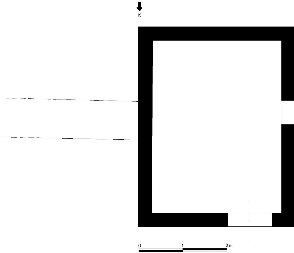
Görsel 16. Hatıplı Değirmeni Planı
