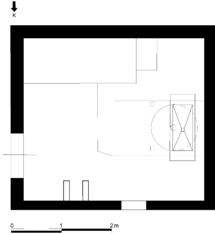
Görsel 8. Hendenli Değirmeni Planı
