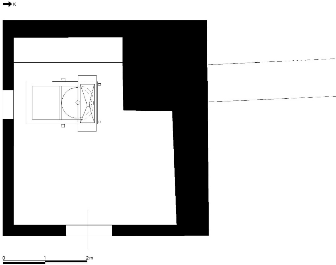
Görsel 3. Egelli Değirmeni Planı
