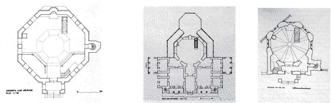
Görsel 21-22-23. İstanbul/Fatih/Orta (Ahmediye) Camii; İstanbul /Fatih/Hırka-i Şerif Camii; İstanbul/Fatih/ Keçecizade Fuat Paşa Camii (soldan sağa) (Ögel, 1989)
