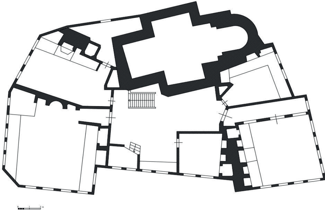
Görsel 2. Haznedaroğlu Konağı Kat Planı (Hanife Kahraman'danışlenerek çizilmiştir) Köşk Bölümü (Seyir Alanı)
