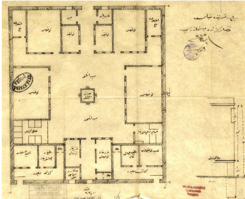
Görsel 7. Darıdere Hapishanesi Projesi ve Kadın Koğuşları (BOA. DH. MB. HPS. M. 1/11)
