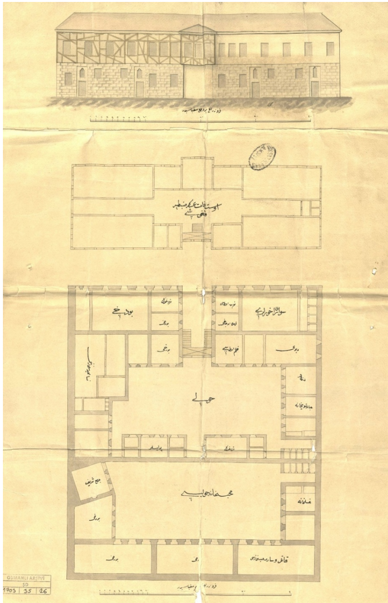
Görsel 15. 1873 Tarihli Konya Hapishane Projesi (BOA. ŞD. 1703/35)
