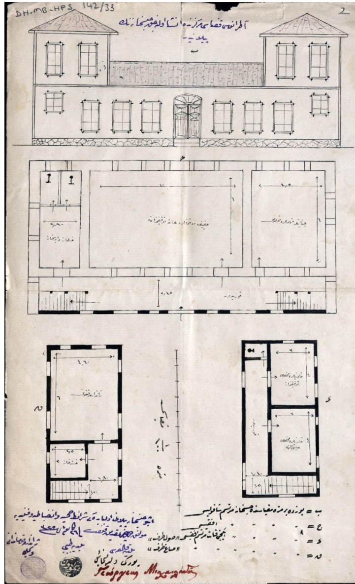
Görsel 14. Atranos Hapishane Projesi (BOA. DH. MB. HPS. 142/33)
