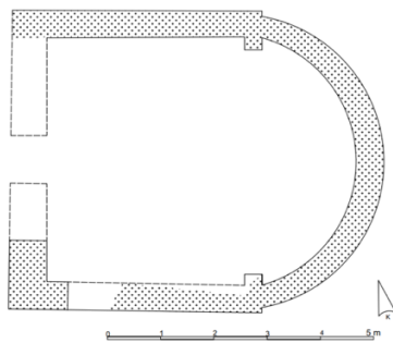
Görsel 6. Aziz Nikolaos Kilisesi Planı (Köse, 2025)
