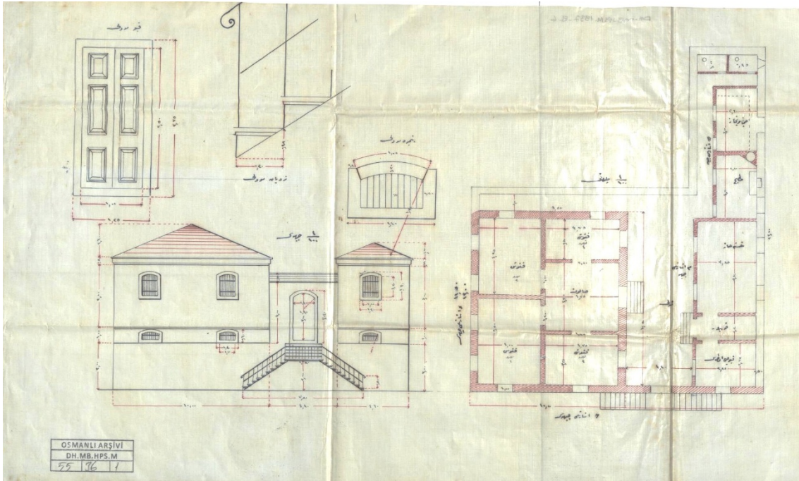
Görsel 8. Aydın Nisa Hapishanesi Projesi (BOA. DH. MB. HPS. M. 55/36)
