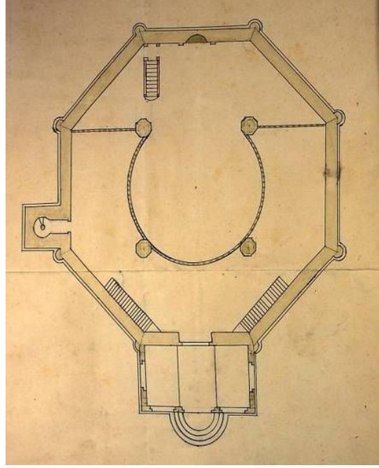
Görsel 24. Batum Aziziye Camii'nin Hacı Dimitri Kalfa tarafından çizilen planı (BOA. MVL 708/110)
