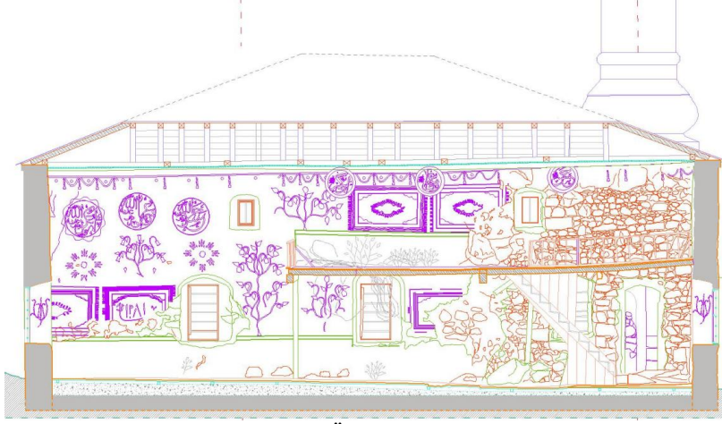
Görsel 17. Batı Duvarı Üzerindeki Süsleme Programının Çizimi
