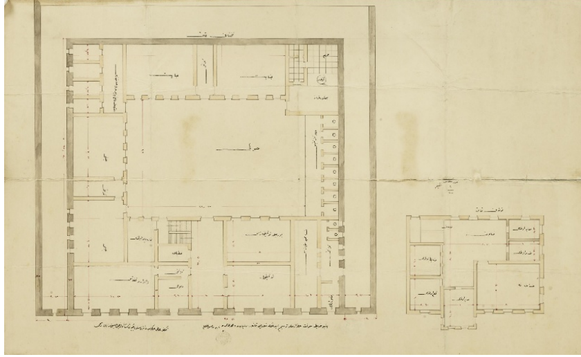
Görsel 6. Tekfurdağı (Tekirdağ) Hapishane Projesi ve Nisa Hapishanesi (BOA. PLK. p. 33/1)
