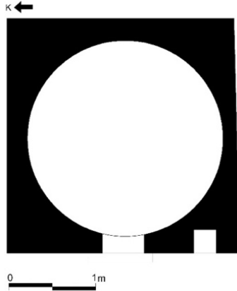
Görsel 42. Havize Çayan Fırını Planı
