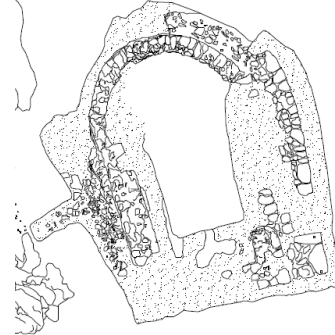
Görsel 6. Aziz Nikolaos Kilisesi Planı (Köse, 2025)
