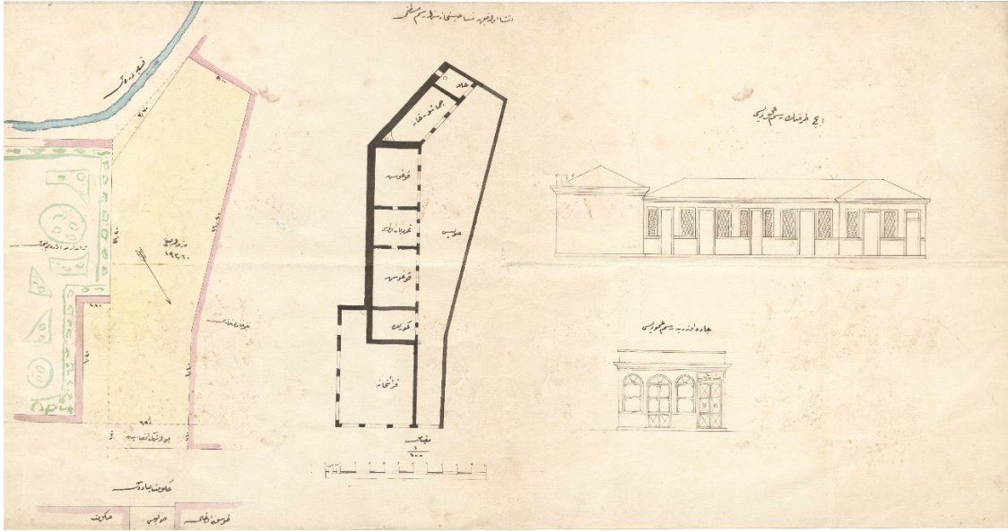
Görsel 11. Anonim bir nisa hapishanesi projesi (BOA. PLK.p 4423)
