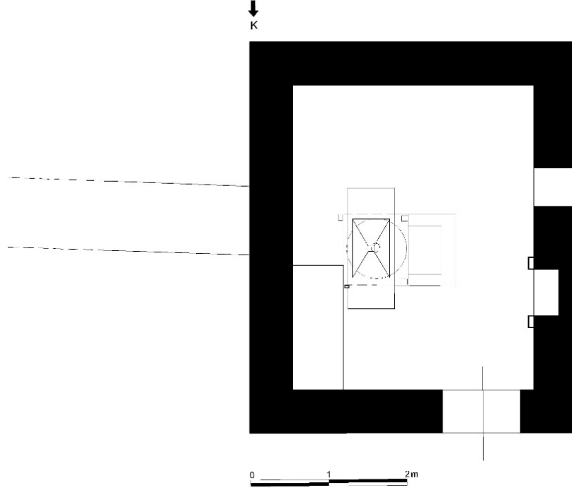
Görsel 11. Pıdırıcı Değirmeni Planı
