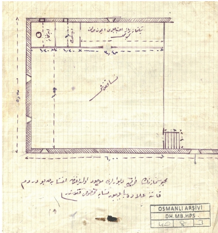
Görsel 1. Fatsa Hapishanesi’nin bodrum katına eklenecek olan Nisa Koğuşu Projesi (BOA. DH. MB. HPS. 40/8)
