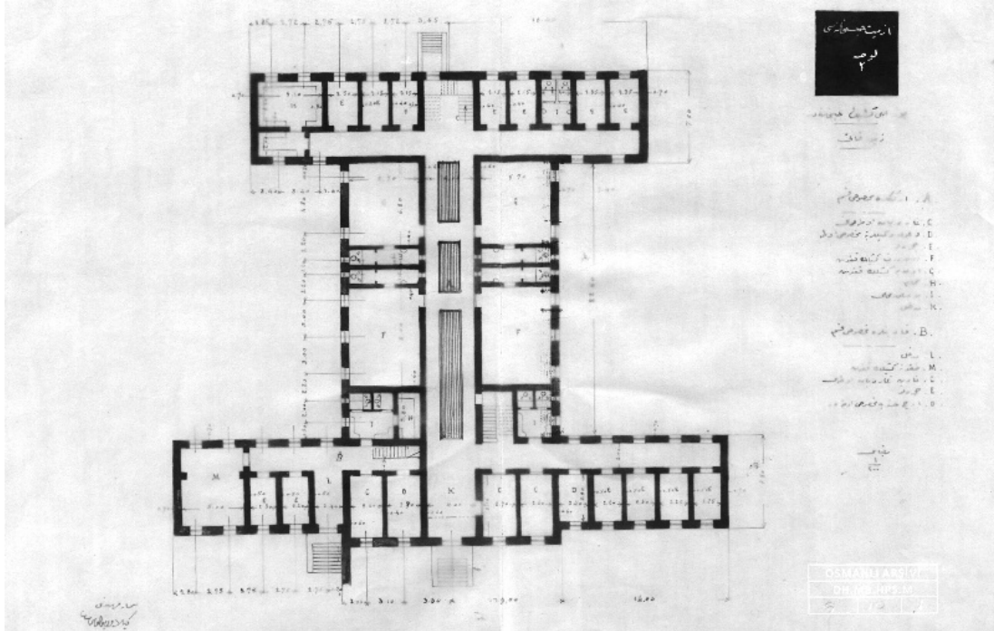
Görsel 4. İzmit Hapishanesi Projesi Zemin Katı ve Kadın Koğuşları (BOA. DH. MB. HPS. M. 5/10)
