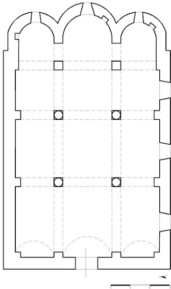
Görsel 1. Muzaras Kilisesi Planı.
