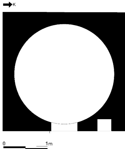
Görsel 37. Mustafa Sevindik Fırını Planı
