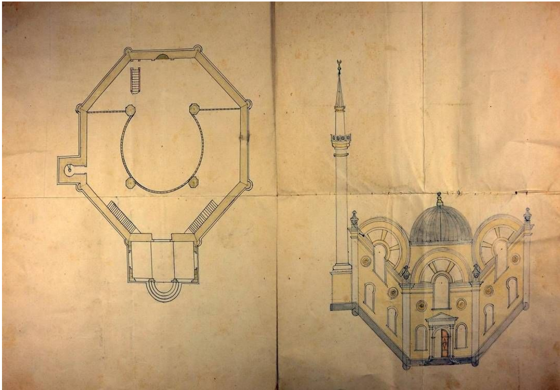
Görsel 15. 1866 yılında Dimitri Kalfa tarafından çizilen Batum Aziziye Cami-i Şerifi'nin plan ve cephe kesiti (Dimitri Kalfa'nın Aziziye Camii için yaptığı ilk çizim (BOA. MVL 708/110).
