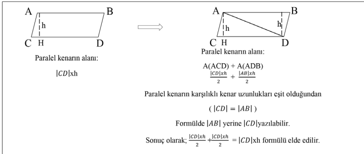
Şekil 6. Üçgen analogisi
